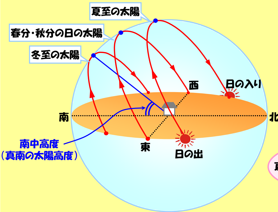
太陽の南中高度の変化(東京)
