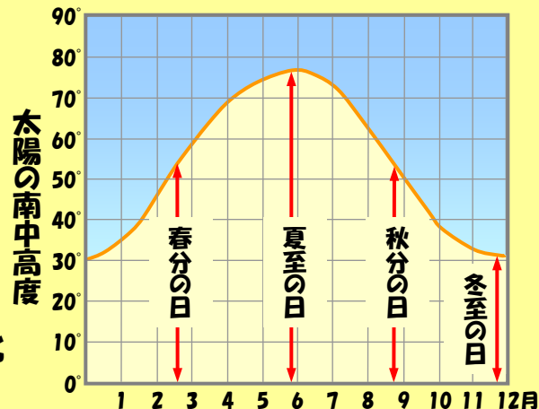
太陽の南中高度の変化(東京)
